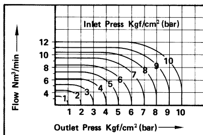
● 流體：空氣 AD-50(AF)
