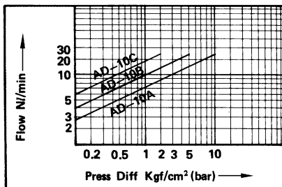
● 流體：液體 AD-10A . 10B.10C
