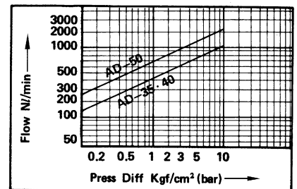
● 流體：液體 AD-35.40.50(AF)
