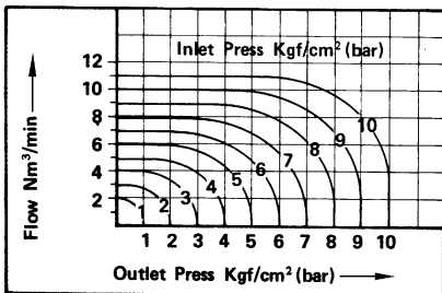
● 流體：空氣 AD-35.40(AF)
