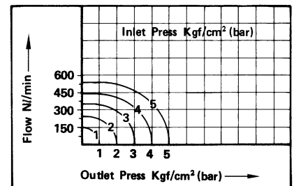
● 流體：空氣 AD-10C . 12B
