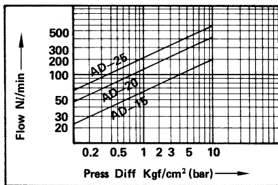
● 流體：液體 AD-14.15.20.25 (AF)
