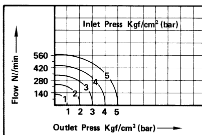
● 流體：空氣 AD-20
