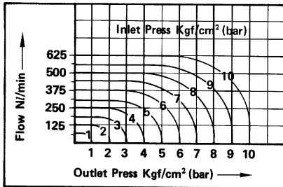
● 流體：空氣 AD-10A
