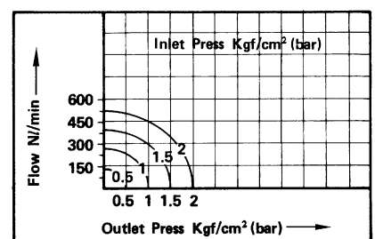
● 流體：空氣 AD-25 (AF)
