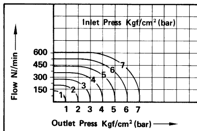
● 流體：空氣 AD-10B . 12A
