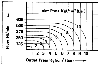
● 流體：空氣 ADS-10A
