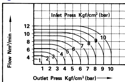
● 流體：空氣 ADS-50(AF)
