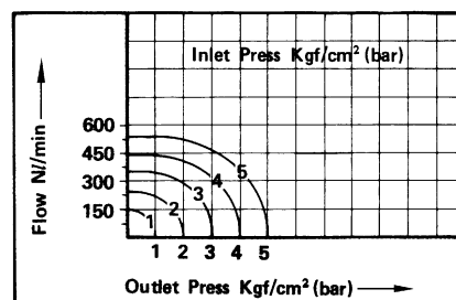
● 流體：空氣 ADS-10C . 12B
