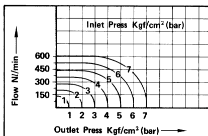
● 流體：空氣 ADS-10B . 12A
