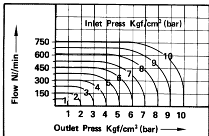
● 流體：空氣 ADS-14.15
