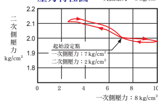
壓力特性圖
