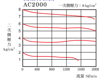
流量特性圖
